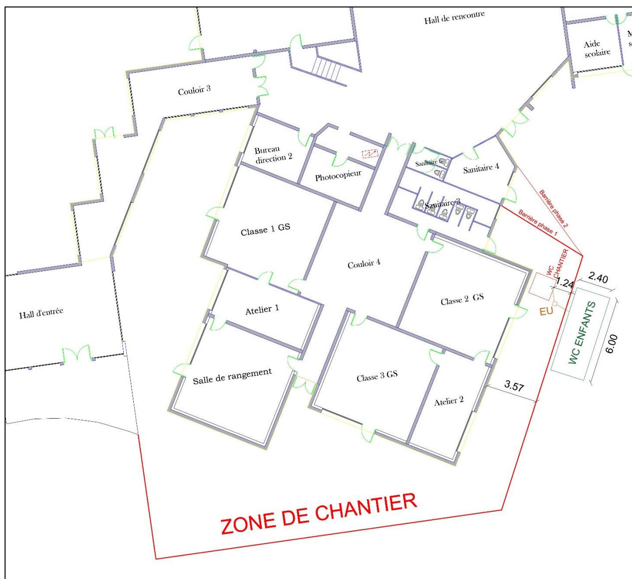
Figure 3 Installation de chantier PHASE 2 et positionnement des sanitaires provisoires dans la cour jusqu'à la fin du chantier.
